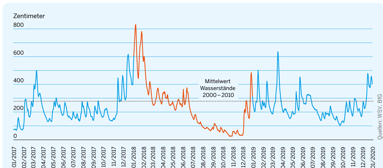
Abbildung 31 Rheinpegel in Düsseldorf bei Rheinkilometer 744,2 für die Jahre 2017 bis 2019
